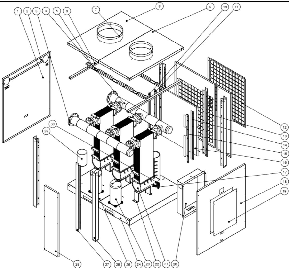
Figure 2 : Composants (indiqués : EVO-RD 7200)
